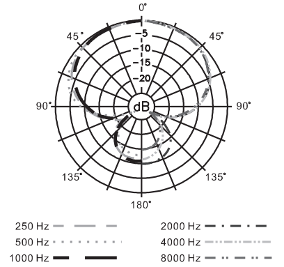
Q6 POLAR PATTERN
